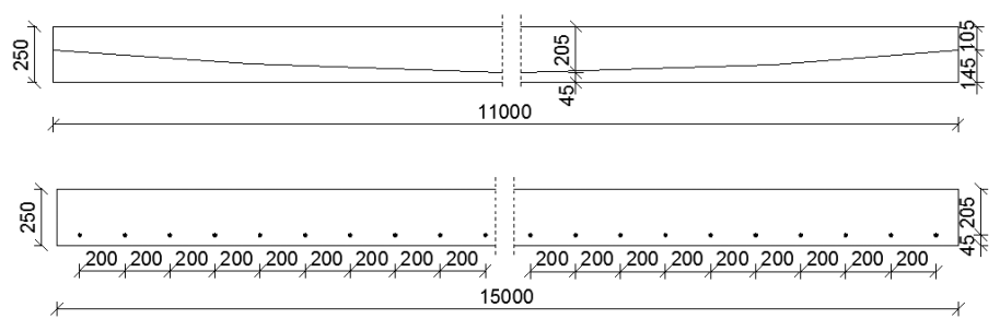
Rys. 6 Geometria i schemat rozmieszczenia kabli w płycie
